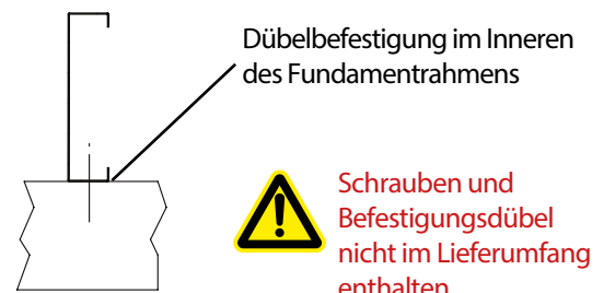
Detail A-A
